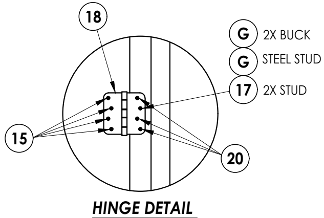
STRIKE JAMB
